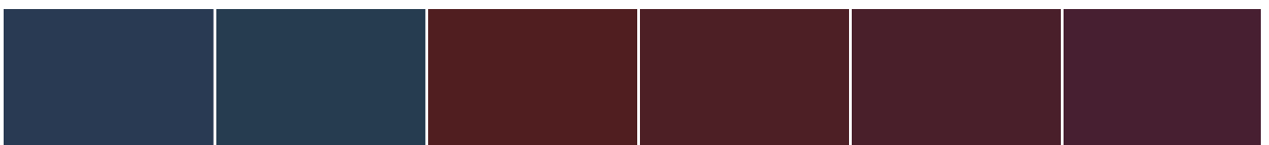
S 4020-R80B
