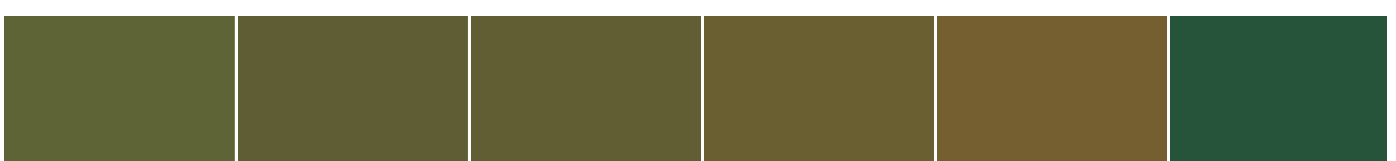
S 3020-G50Y
