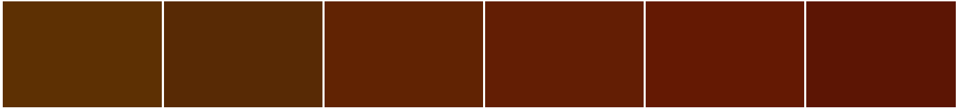
S 3560-Y
