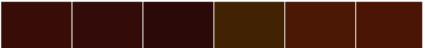
S 5040-Y70R
