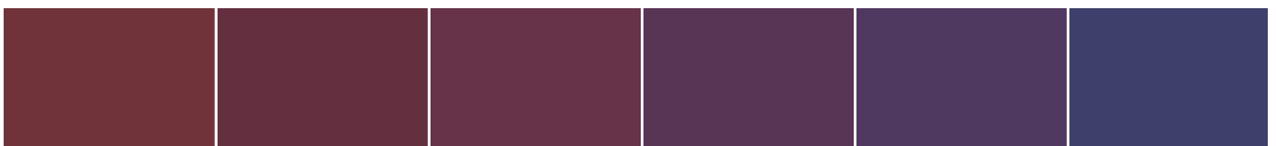
S 3030-R10B
