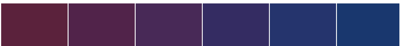
S 3040-R30B
