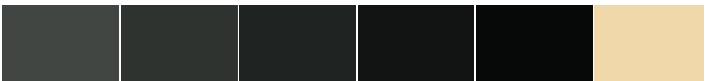
S 4502-G
