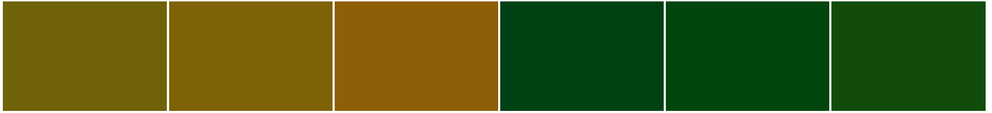
S 2060-G70Y
