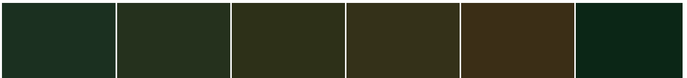
S 5020-G10Y
