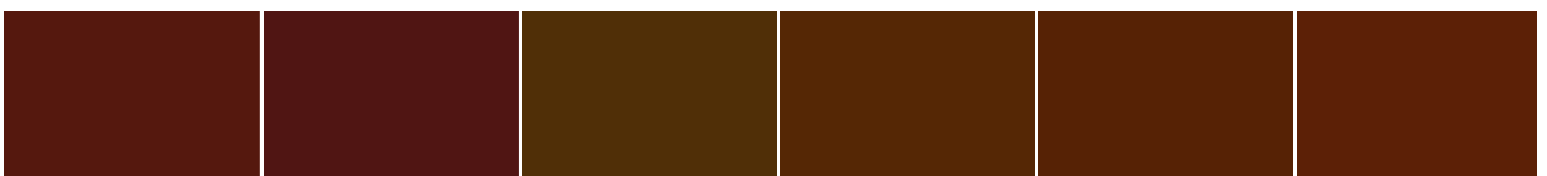
S 4040-Y70R
