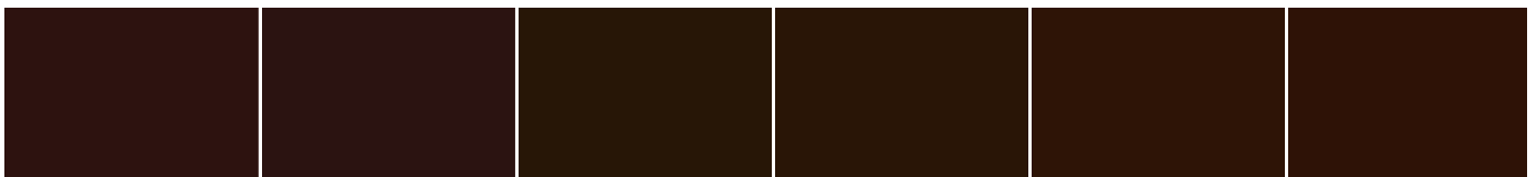
S 6020-Y80R
