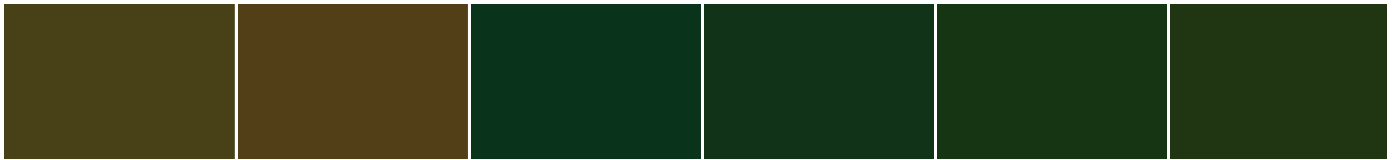
S 4030-G70Y
