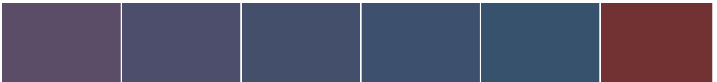
S 3020-R50B
