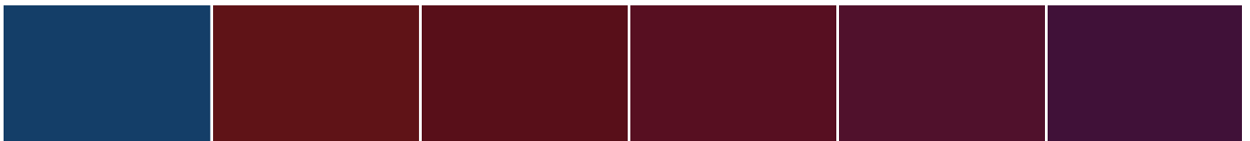
S 3040-R90B
