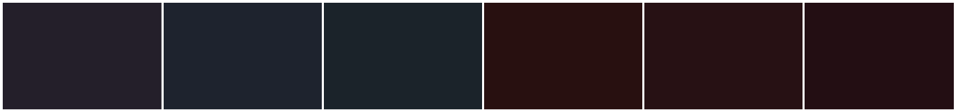
S 6010-R50B
