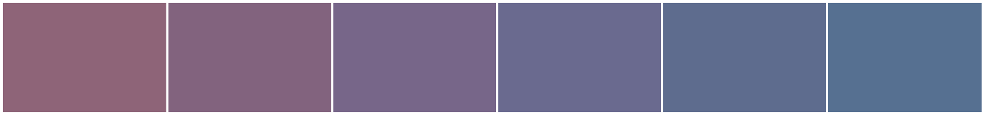
S 2020-R30B
