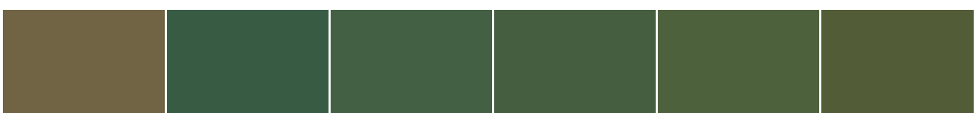
S 3010-G90Y
