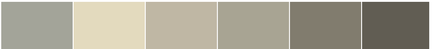
S 1502-G50Y
