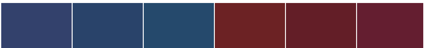
S 3030-R70B
