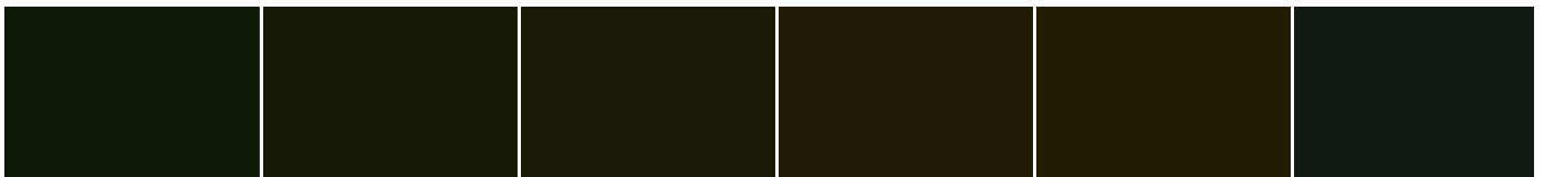
S 5540-G30Y
