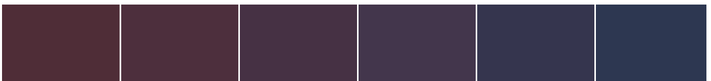
S 4020-R20B
