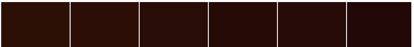
S 6030-Y40R
