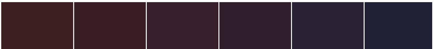
S 5020-R10B
