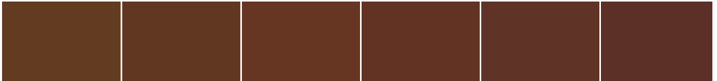
S 4020-Y30R
