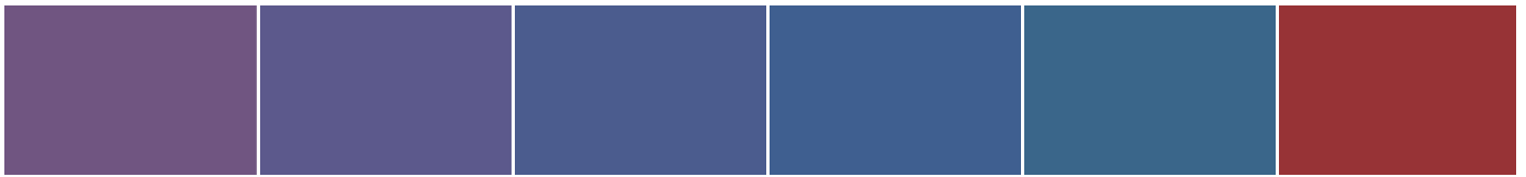
S 2030-R50B
