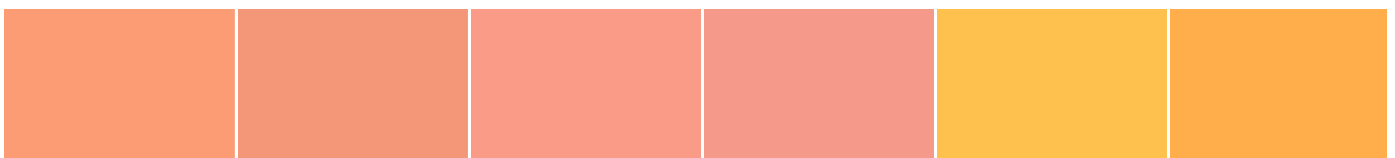
S 0520-Y60R
