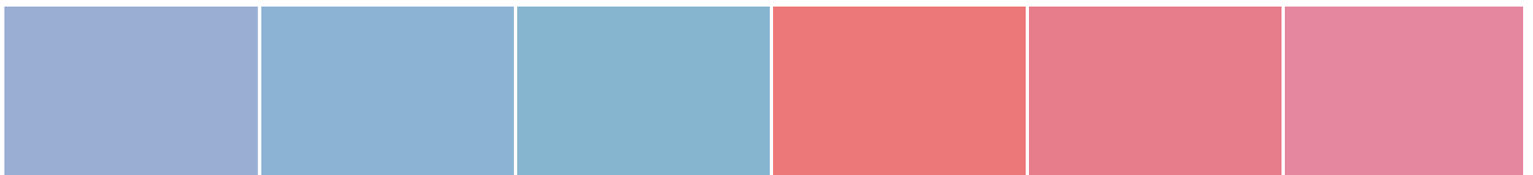
S 0520-R70B
