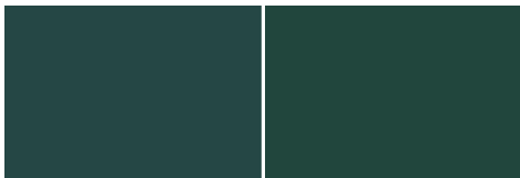
S 4020-B50G
