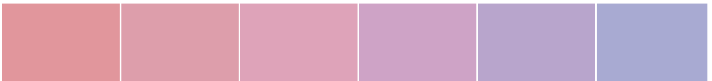
S 0520-R10B
